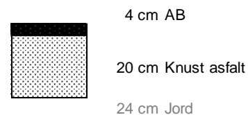
Figur 3 Alternativ med ét lag asfalt og knust asfalt (T0 = Kun lette køretøjer)
