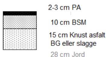
Figur 5 Alternativ med ét lag asfalt på BSM
