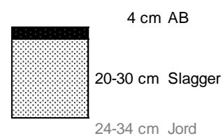
Figur 4 Alternativ med ét lag asfalt og slagger (T1 <1 lastbil pr. døgn)
