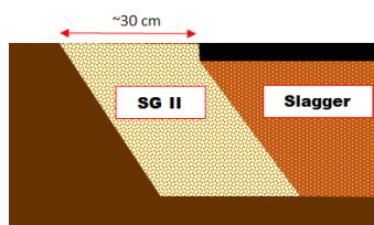
Figur 7 Forslag til udformning af skulder så slaggerne er afdækkede
